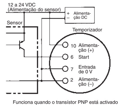
Funciona quando o transistor PNP está activado
