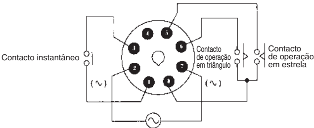
H3CR-G8EL
