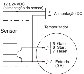
Funciona quando o transistor está activado
