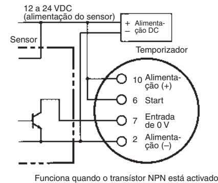
Funciona quando o transistor NPN está activado
