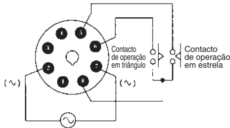
H3CR-G8L
