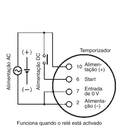
Funciona quando o relé está activado
